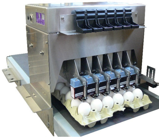
Egg-Jet Sprinter R6, Serie 20, auf Transportband
